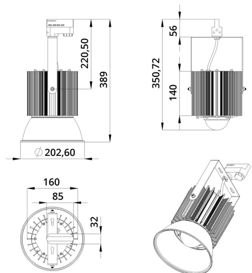
Габаритный чертеж
