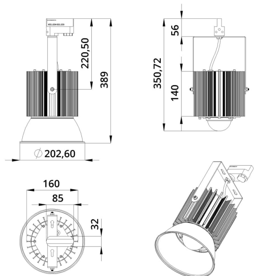
Габаритный чертёж
