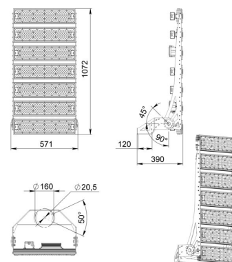
Габаритный чертёж
