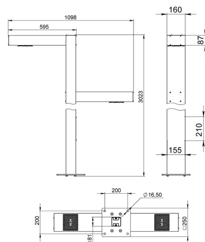
Габаритный чертеж
